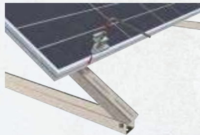
Paneelien asennus mahdollista myös ilman profiilikiskoa
