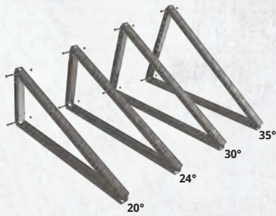
Monipuoliset asennuskulmat 20–45 (astetta)
