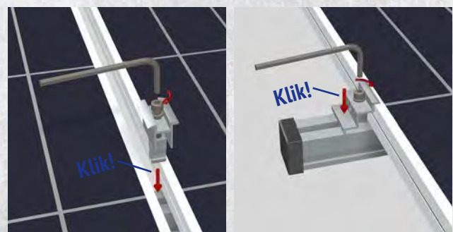
Nopea paneelin kiinnitys
