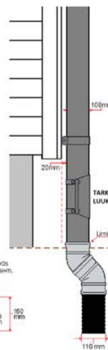
SUORA LIITOS VIEMÄRIPUTKEEN, OHJAUS / KOHDISTUS TÄYTÖN ALLA.
