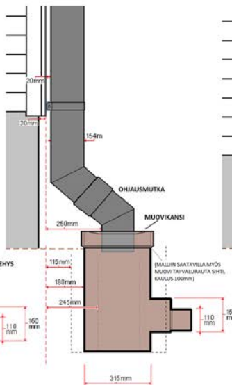
OHJAUSMUTKALLA KAIVON SISÄÄN, YLEENSÄ UMPIKANNEN LÄPI, KAIVOMALLI SYVÄ, KANSI AVATTAVISSA.
