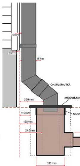
OHJAUSMUTKALLA KAIVON SISÄÄN, UMPIKANNEN LÄPI, KAIVOMALLI SYVÄ, KANSI AVATTAVISSA.
