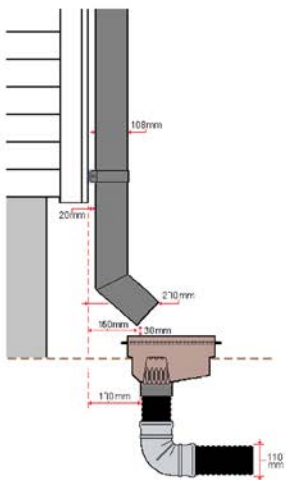
ULOSHEITOLLA RÄNNIKAIVOON
